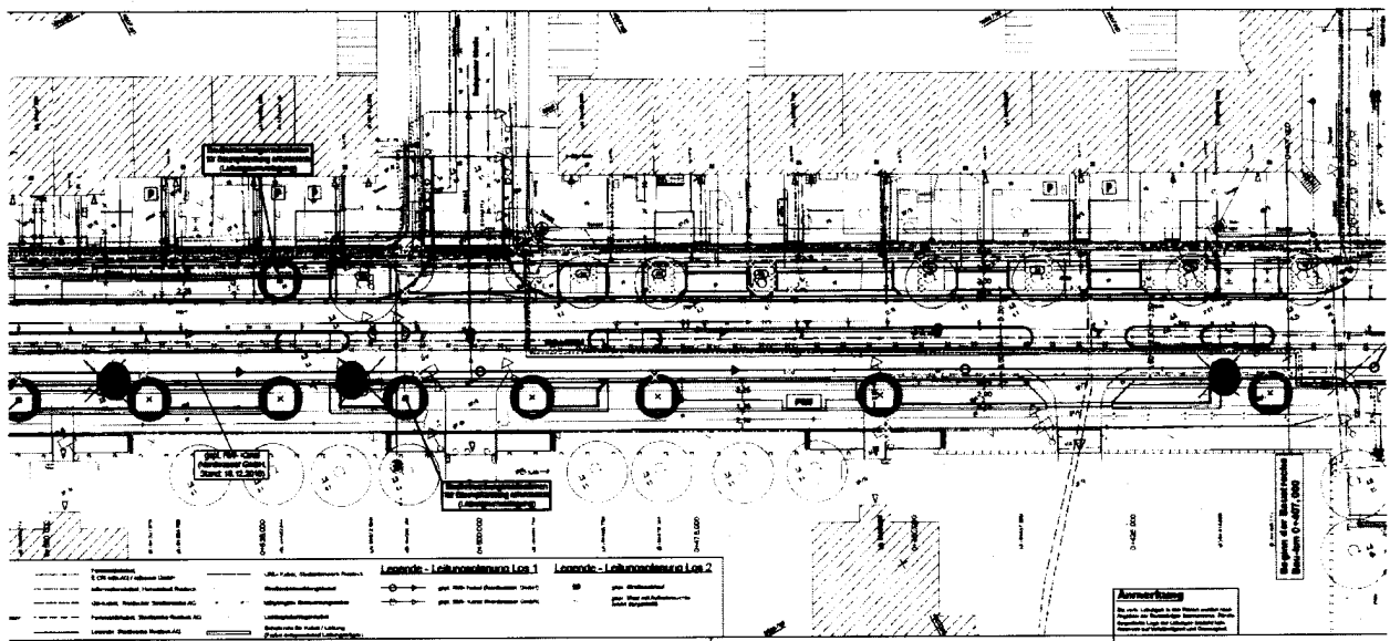
Auszug aus der Genehmigungsplanung
